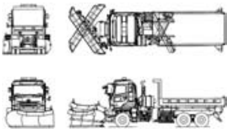
除雪トラック（雪寒機械）外觀図
