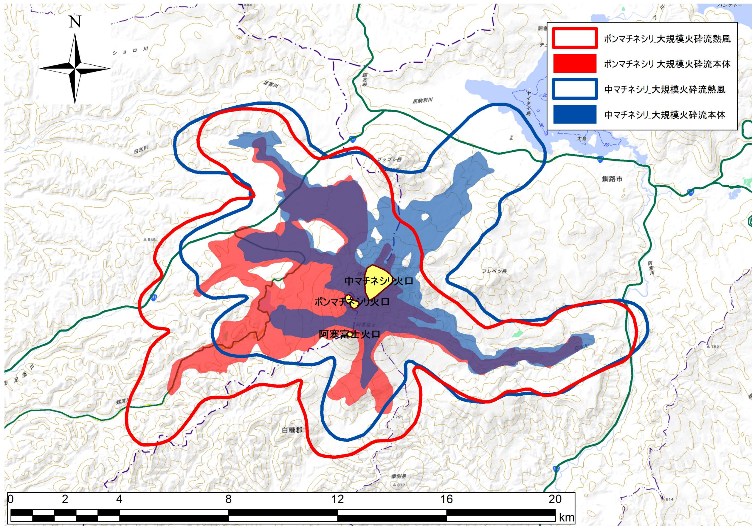
図 6 噴火火口ごとの火砕流・火砕サージ影響範囲
