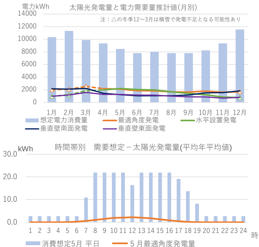
図 6.5 事業所 20kW 太陽光設置発電量推計
