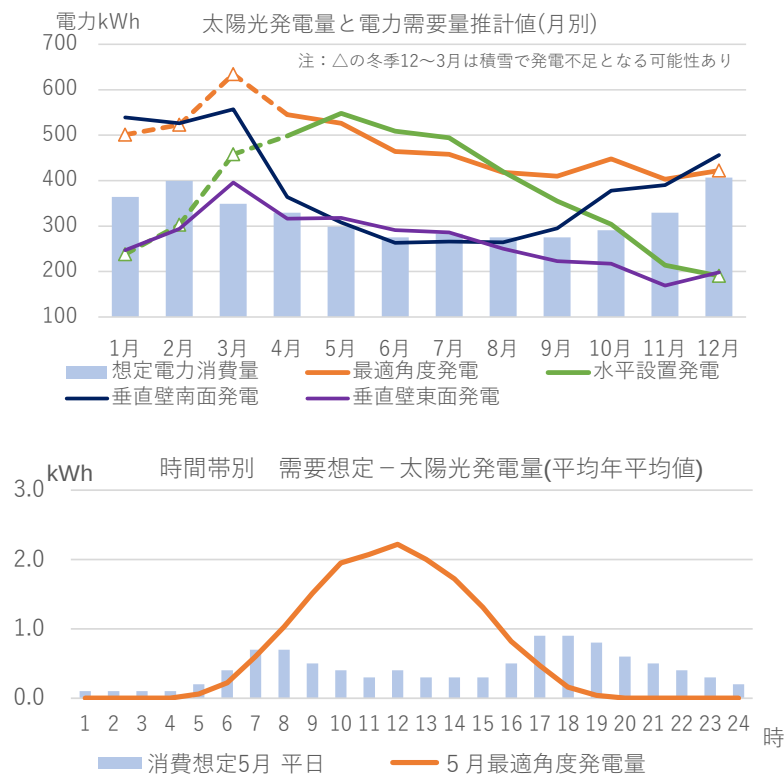
図 6.4 戸建住宅 5kW 太陽光設置発電量推計
