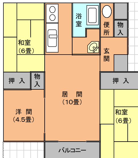
(6) 東団地 1026 号室 (2 階・3LDK)
