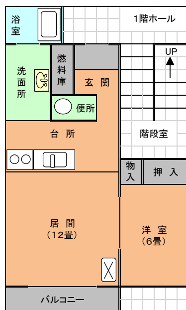
(5) 東団地 1016 号室 (1 階・1LDK)
