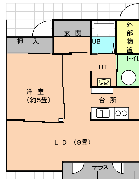
(25) はるにれ団地 904 号室 (平屋・1LDK)
